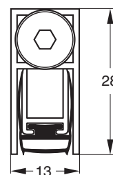
Stribo Acoustic Plus Fin
